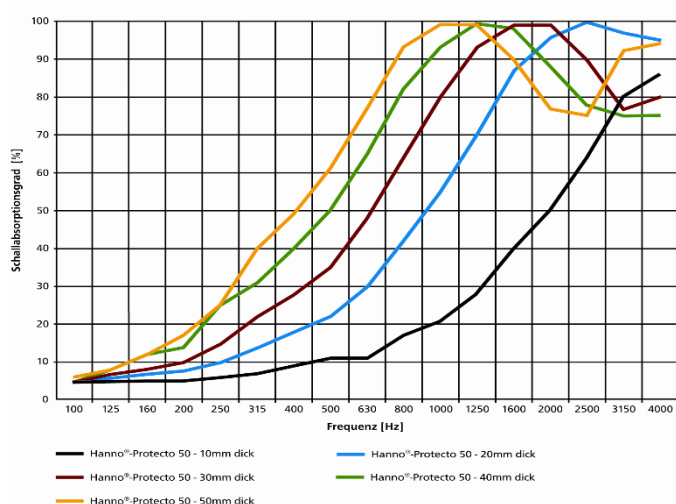
Messung nach DIN-EN-ISO 10534-2 Impedanzrohr
